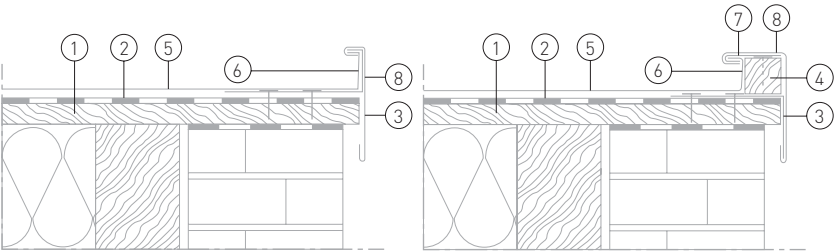
Verge, no batten
